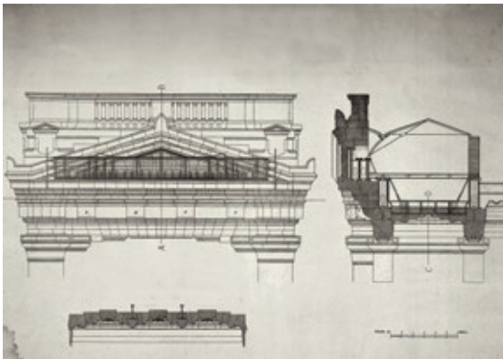
Natuursteen en metaal vermengd en samenwerkend als één constructie om grote overspanningen te kunnen realiseren, een meesterwerk van ingenieur François Wellens.
